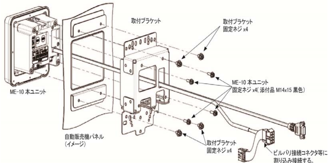
自販機取付例
